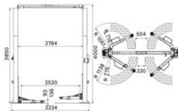
350.40 - טון 4
